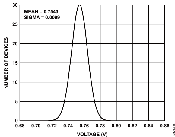
图7. 范围2直流偏置分布, VDD = 3.3 V
