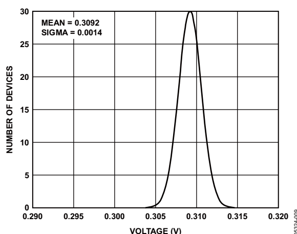
图9. 范围3直流偏置分布, VDD = 3.3 V
