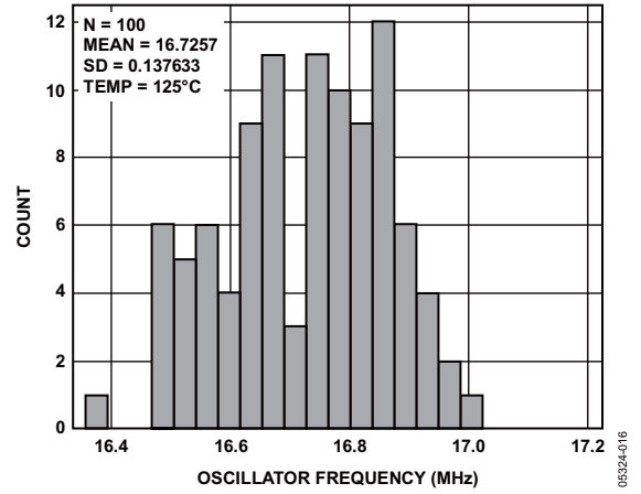
图16. 125°C时内部振荡器的频率分布
