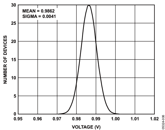
图6. 范围2输出激励电压分布, VDD = 3.3 V
