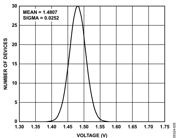
图5. 范围1直流偏置分布, VDD = 3.3 V
