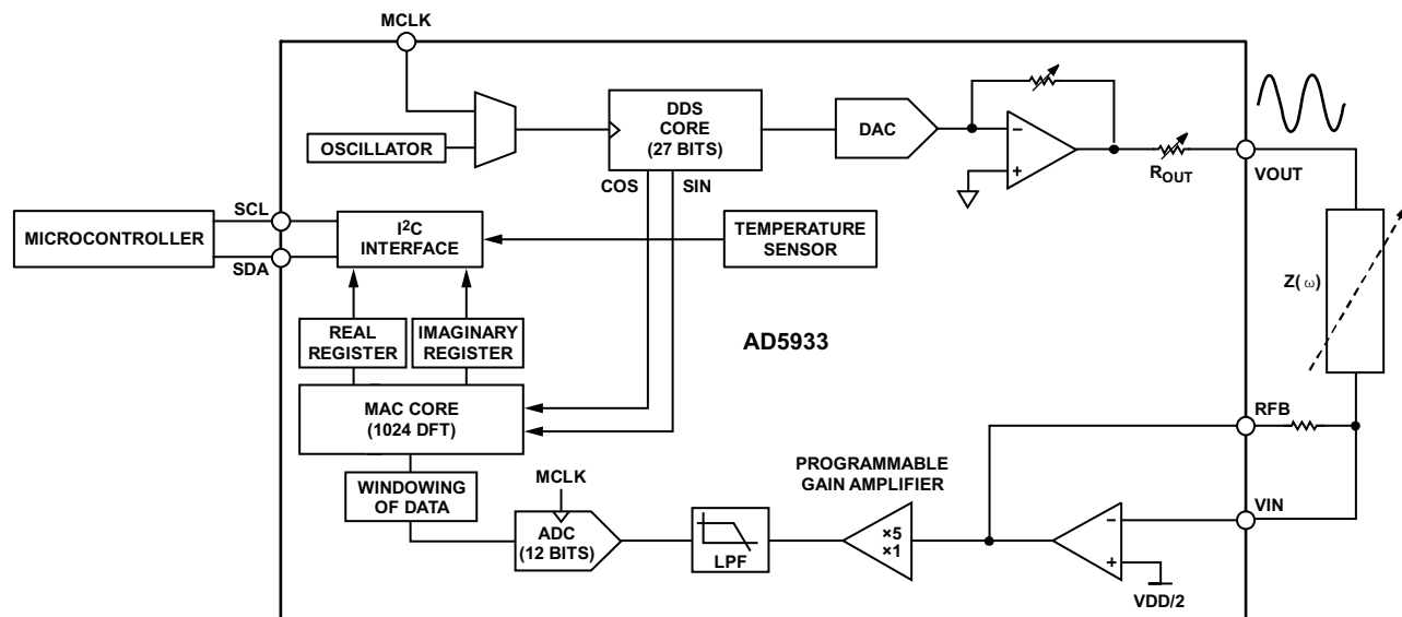
图17. 功能框图
