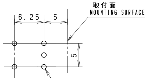
端子取付穴寸法図 (挿入側より見た図) (許容差±0.1) 5 - φ1 +0.1 穴 HOLES
