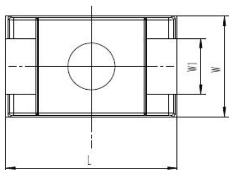
底部视图
