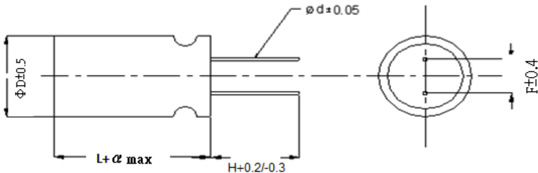
Fig. 2 Dimension
