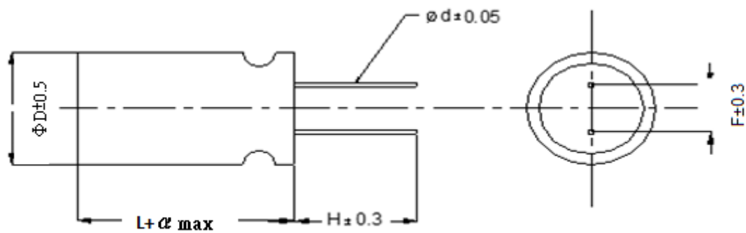
Fig. 2 Dimension
