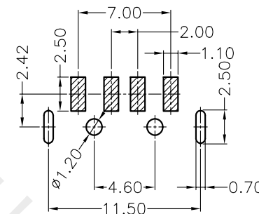
P.C.B LAYOUT(TOL:±0.05)
