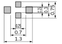
NFM15CC/15PC
