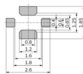
NFM21PS
