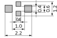
NFM18CC/18PC
