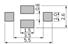
NFM41CC/41PC
