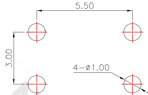
PCP Layout(Pattern Side)
