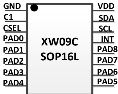
芯片引脚图
