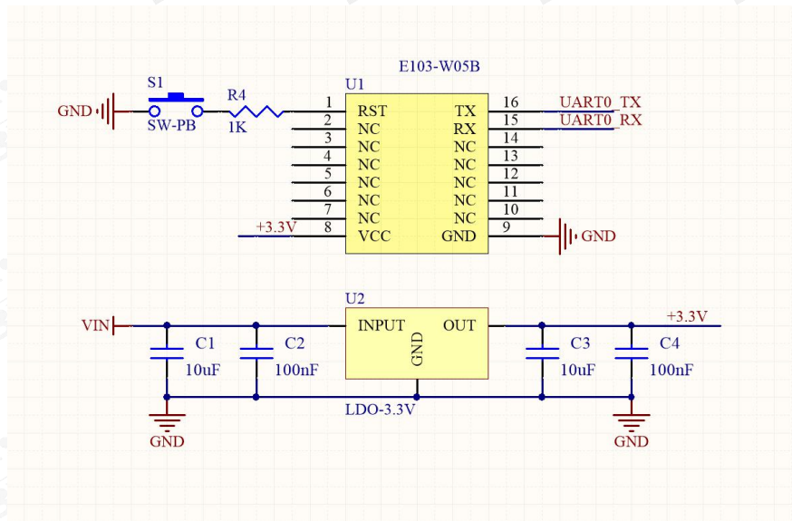
图 5-1 电路图
