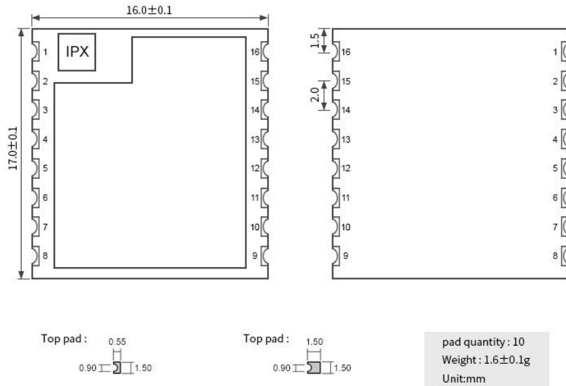
图 3-1 机械尺寸与引脚定义
