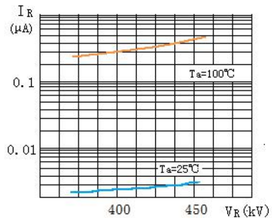
反向特性曲线 (2CL450KV/1A) Reverse Characteristics
