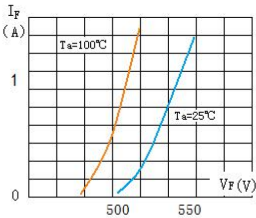
正向特性曲 (2CL450KV/1A) Forward Characteristics
