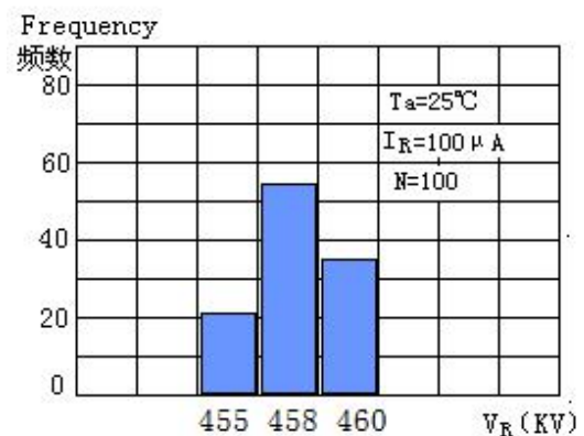
反向雪崩电压分布 (2CL450KV/1A) Avalanche Breakdown Voltage Distribution
