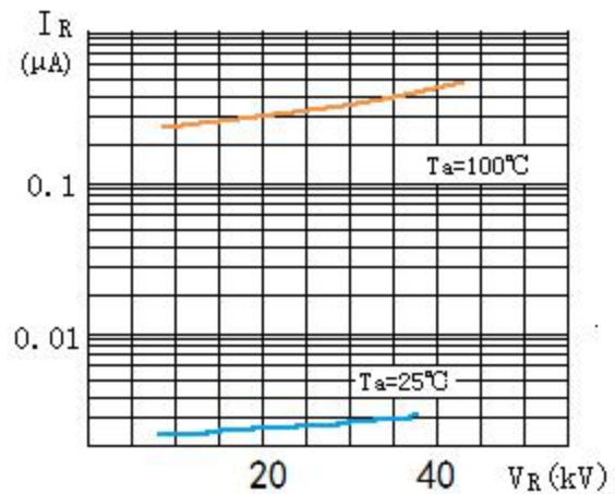
反向特性曲线 ( 2CL35KV/3A ) Reverse Characteristics
