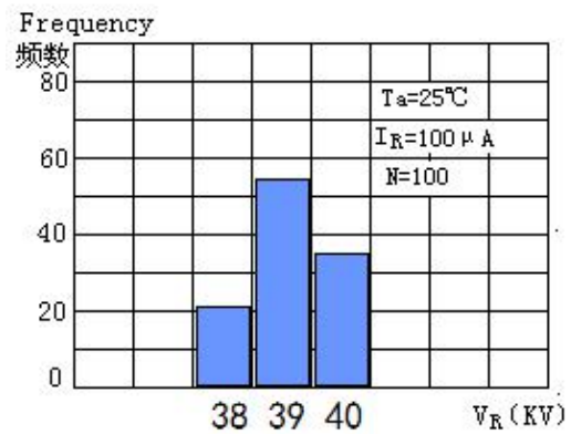
反向雪崩电压分布 ( ( 2CL35KV/3A ) Avalanche Breakdown Voltage Distribution
