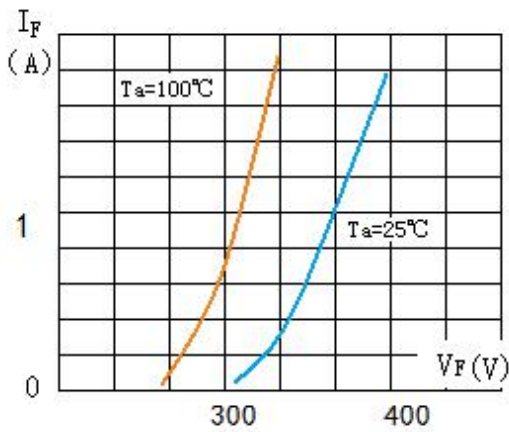
正向特性曲 ( 2CL300KV/1A ) Forward Characteristics
