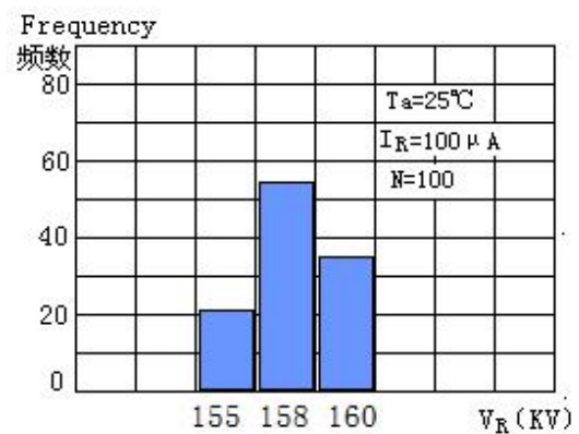
反向雪崩电压分布 ( 2CL150KV/0.5A ) Avalanche Breakdown Voltage Distribution
