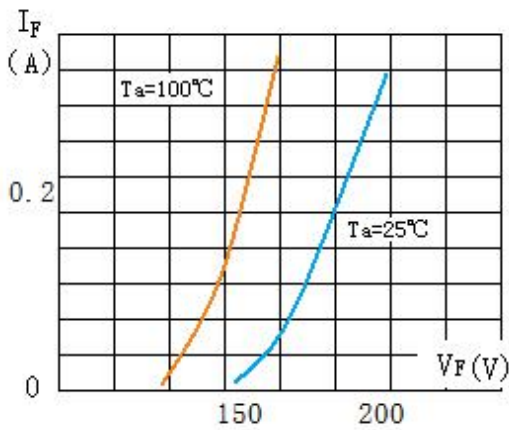
正向特性曲 ( 2CL150KV/0.2A ) Forward Characteristics
