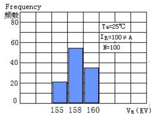
反向雪崩电压分布 ( 2CL150KV/0.2A ) Avalanche Breakdown Voltage Distribution
