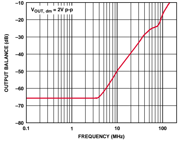
图39. 输出平衡与频率的关系
