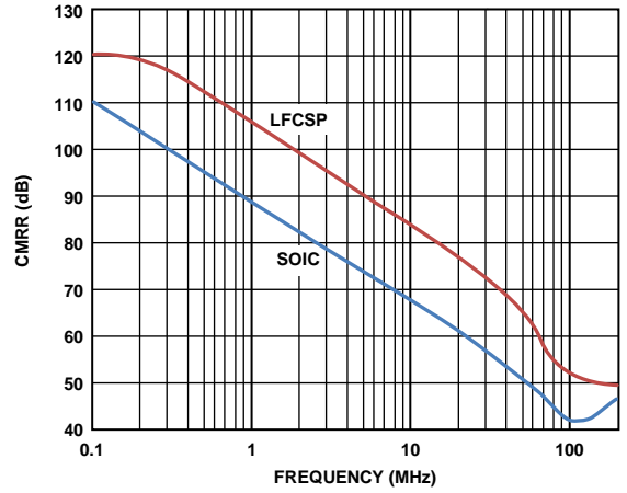
图38. CMRR与频率的关系
