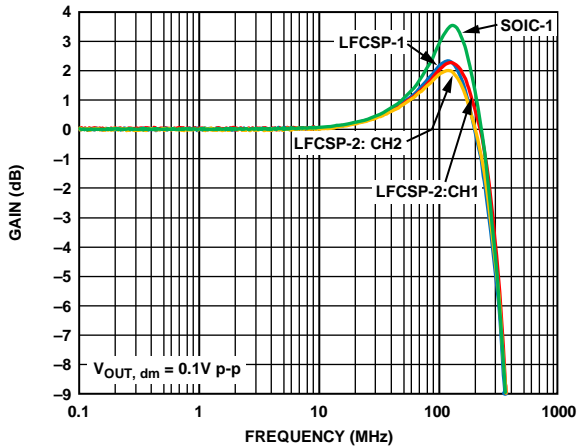
图13. 不同封装下的小信号频率响应
