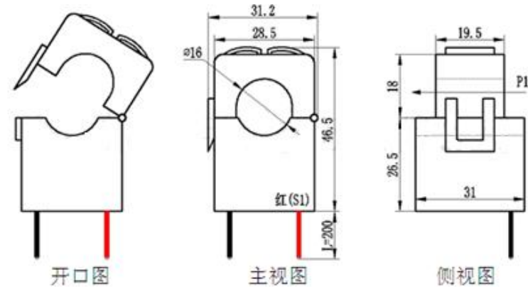
100A 开口式电流互感器外形尺寸图
