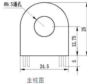
电流互感器外型及尺寸图：
