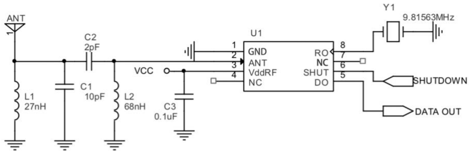
图1 315MHz 1.5kbps典型电路
