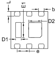
Bottom View 背面视图
