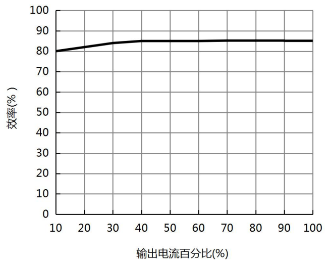
图 6. B0505S-W5R3 效率 vs 输出负载 (标称输入)
