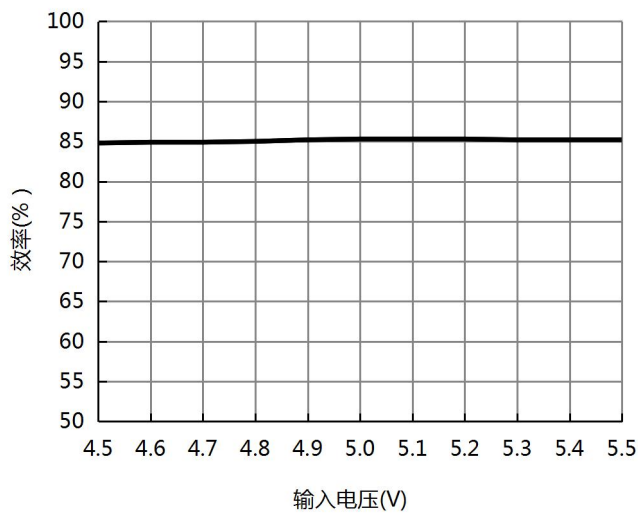
图 5. B0505S-W5R3 效率 vs 输入电压 (满载)
