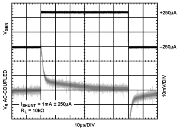
图12. ADR5045 瞬态响应
