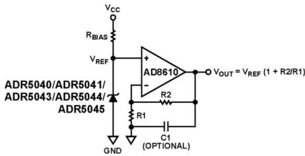
图22. 可调电压源
