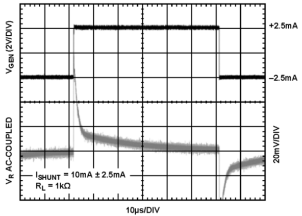
图13. ADR5045 瞬态响应
