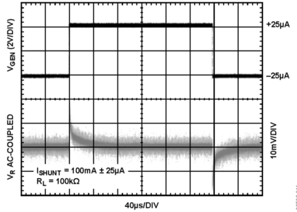
图11. ADR5045 负载瞬态响应
