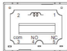
(底视图)
