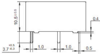
外形图
