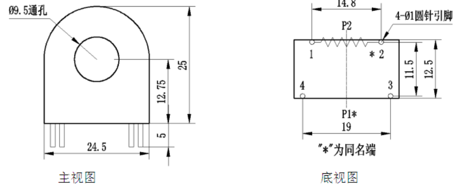
50A 穿心式电流互感器外形尺寸图
