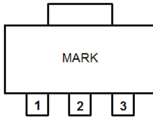
SOT89-3
