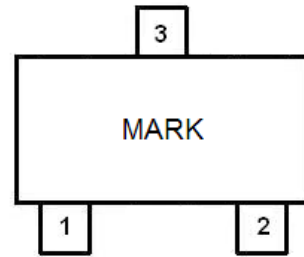
SOT23-3
