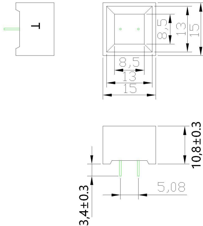
方形平面管 RGB-1515 深绿色 外形图: (Unit:mm Tolerance: \pm 0.3 mm)
