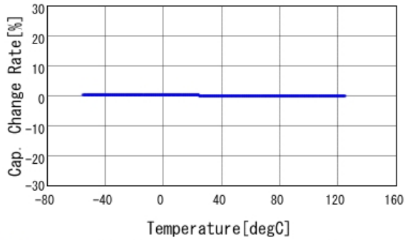
温度特性
