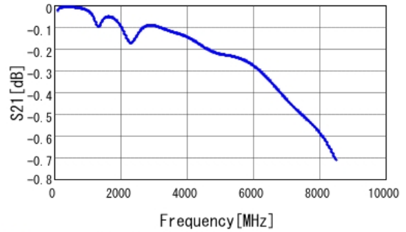
S参数S21
