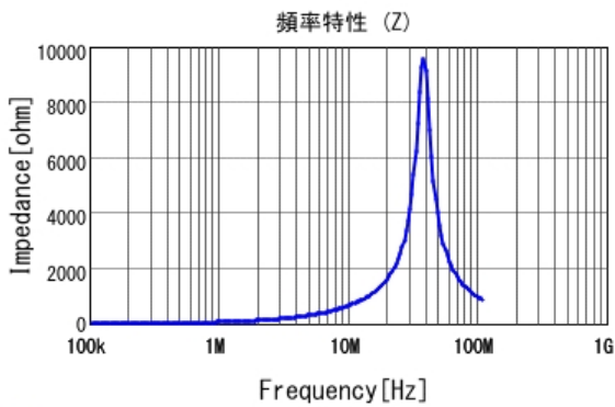
■ LQH3NPZ100MME |Z|
