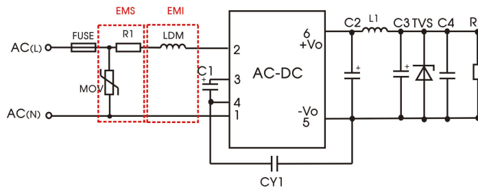
推荐电路 4
