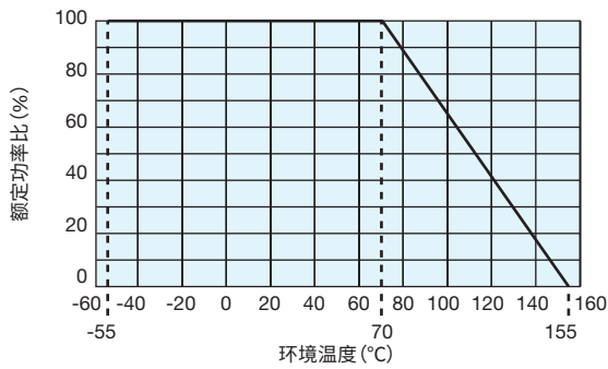
环境温度
