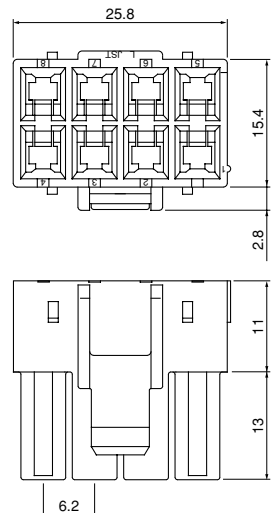
<8 circuits>
