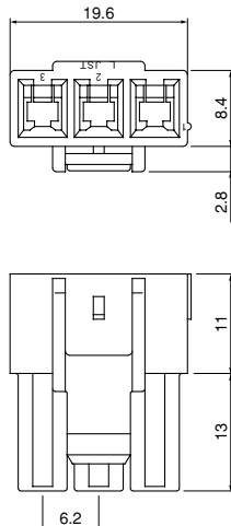
<3 circuits>
