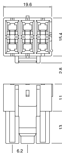
<6 circuits>
