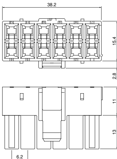
<12 circuits>
