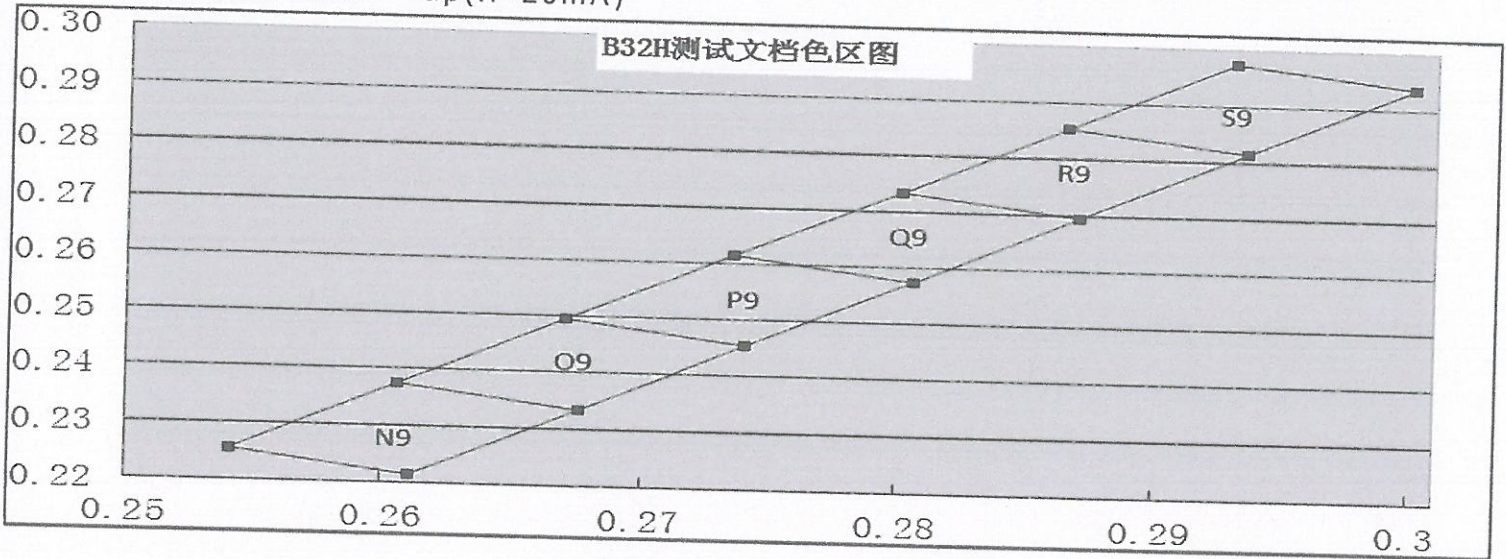
色度坐标分档 Color Bin Code (If=20mA)
