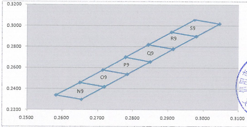
色度坐标分档 Color Bin Code (If=20mA)
