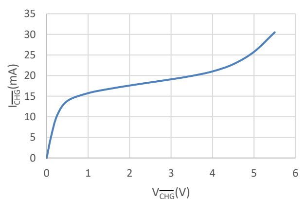
I_{\text{CHG}} vs V_{\text{CHG}}
