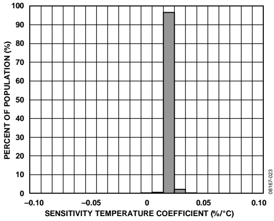
图23. Y轴灵敏度温度系数, V_s = 2.6 V
