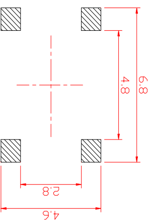
PCB. 焊接图
