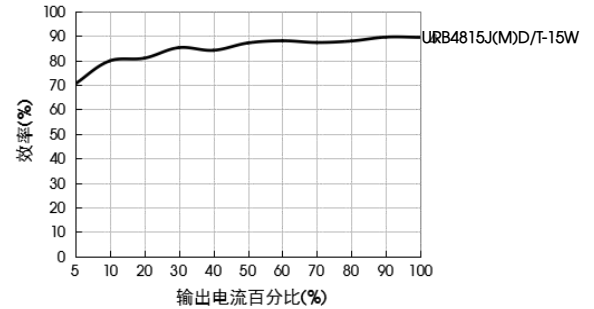
效率Vs输出负载 (Vin=48V)
