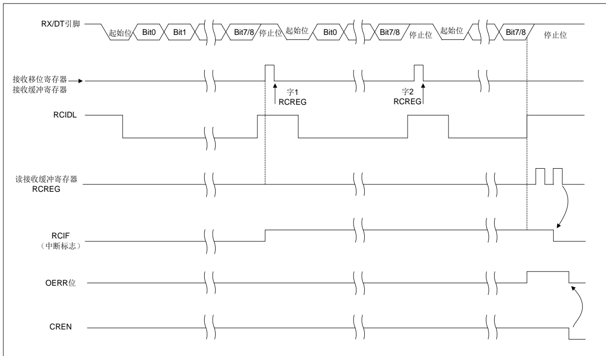
图 14-5: 异步接收
