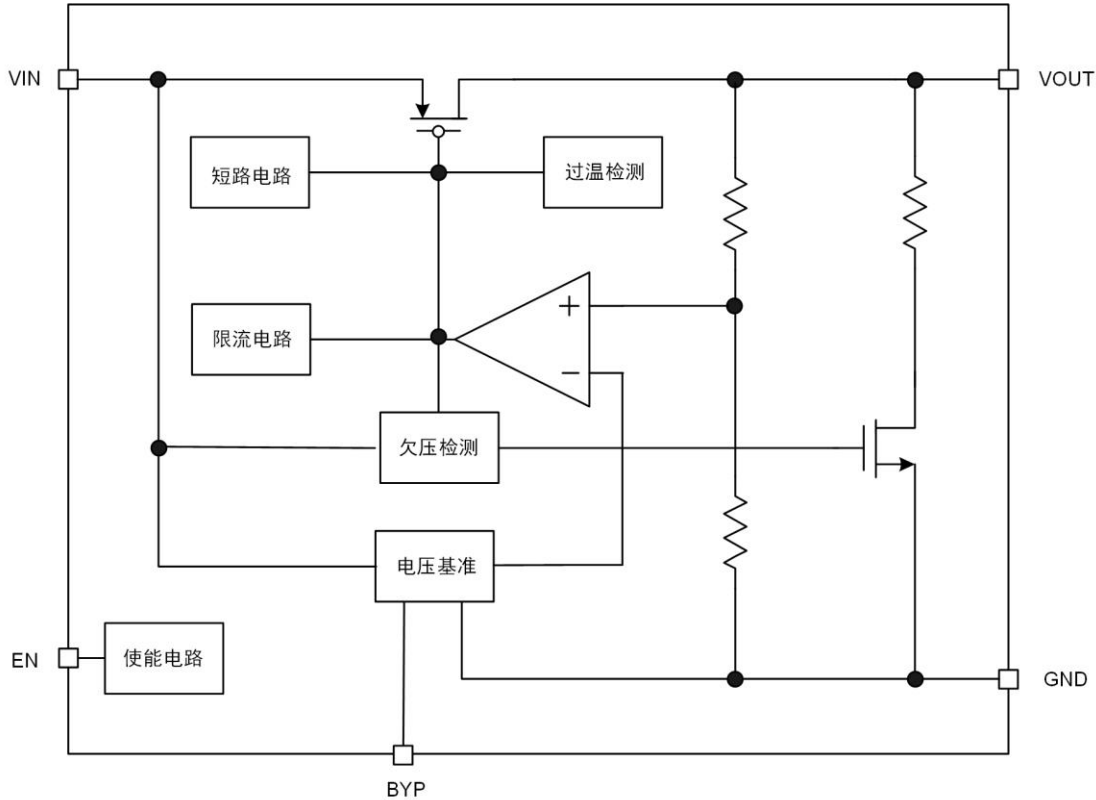
图 3.1 芯片内部框图
