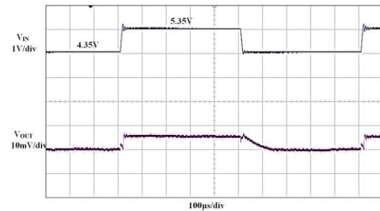
图 2.16 线性瞬态响应波形
