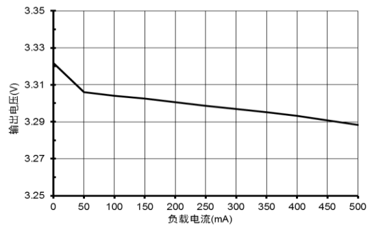
图 2.5 负载调整特性
