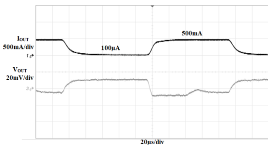
图 2.17 负载瞬态响应波形
