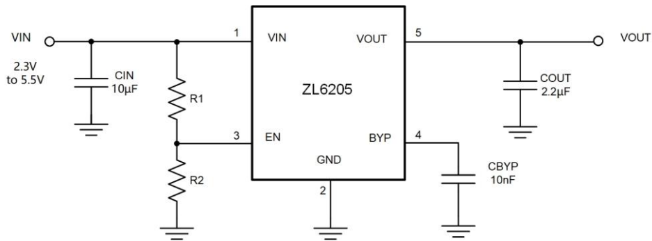
图 4.1 ZL6205 典型应用电路
