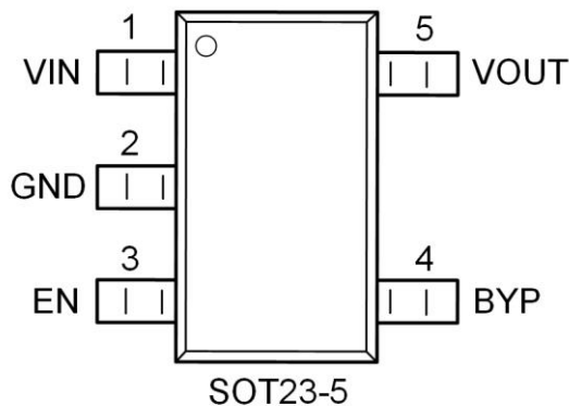
图 2.1 管脚信息
