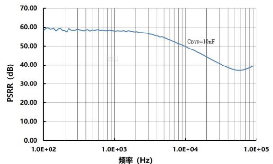
图 2.9 PSRR 与频率的关系 ( I_{OUT}=1mA )
