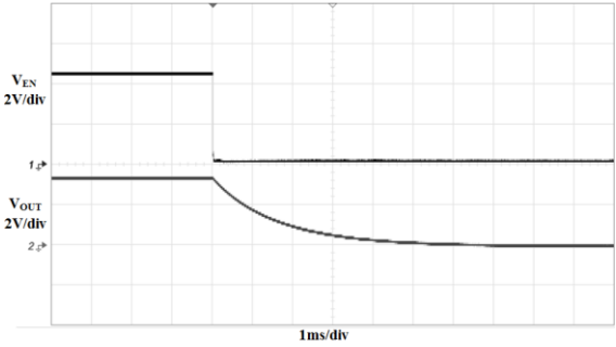
图 2.11 EN 禁能关闭波形(100µA 负载)
