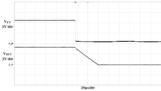
图 2.13 EN 禁能关闭波形(500mA 负载)
