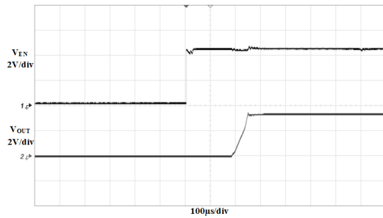
图 2.10 EN 使能启动波形(100µA 负载)
