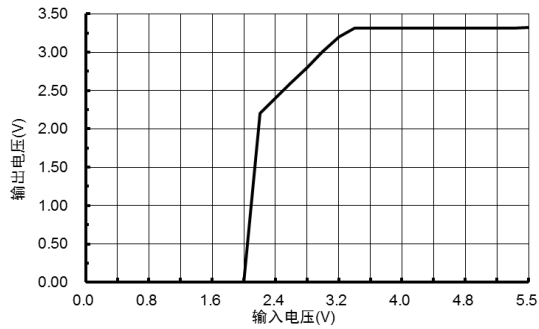
图 2.2 输入输出电压特性
