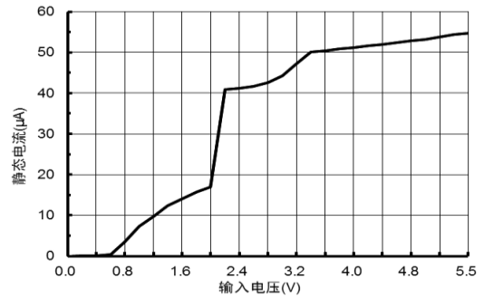
图 2.3 静态电流与输入电压关系
