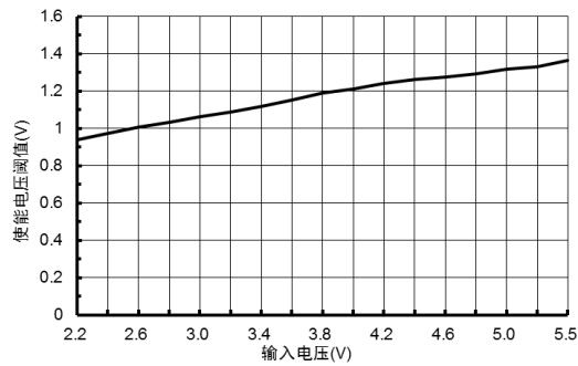
图 2.6 使能电压阈值与输入电压的关系
