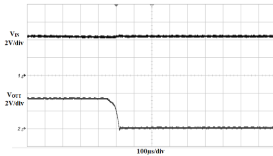
图 2.14 输出短路波形
