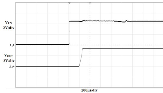
图 2.12 EN 使能启动波形(500mA 负载)
