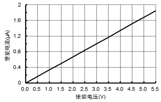
图 2.7 使能电流与使能电压的关系
