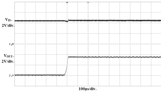
图 2.15 输出短路恢复波形
