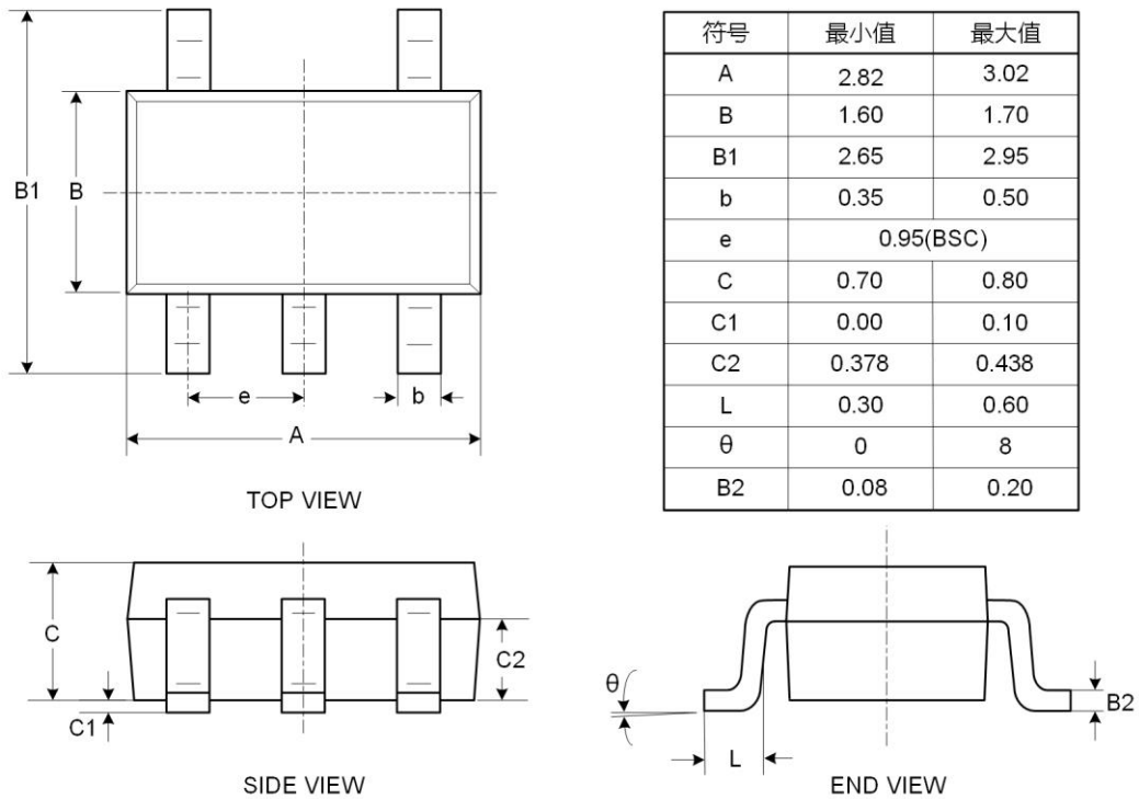
图 5.1 封装尺寸图
