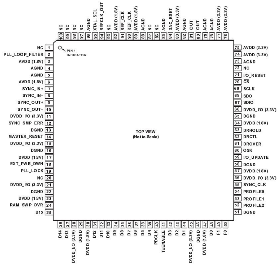
图 2 芯片管脚图
