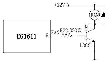
图 8.6a FAN 风扇控制输出
