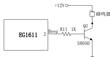
图 8.7a 蜂鸣器控制输出
