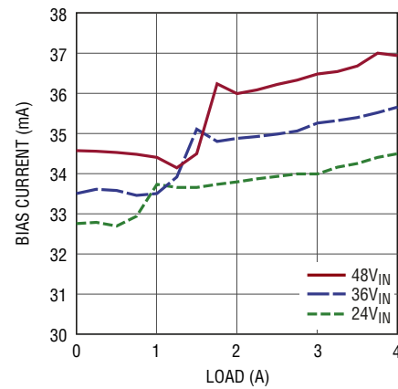
偏置电流与负载的关系曲线， V OUT = 15V
