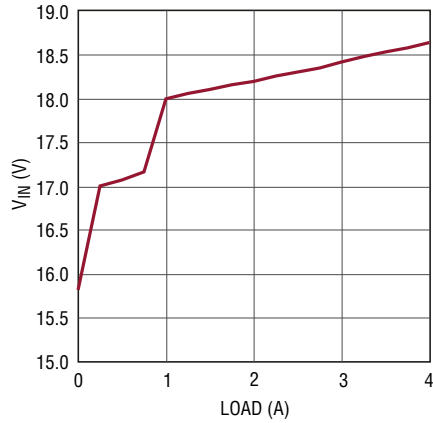
最小 V IN 与负载的关系曲线， V OUT = 15V
