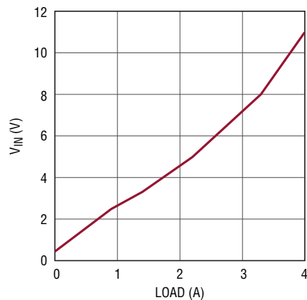
最小 V IN 与负载的关系曲线， V OUT = -5V
