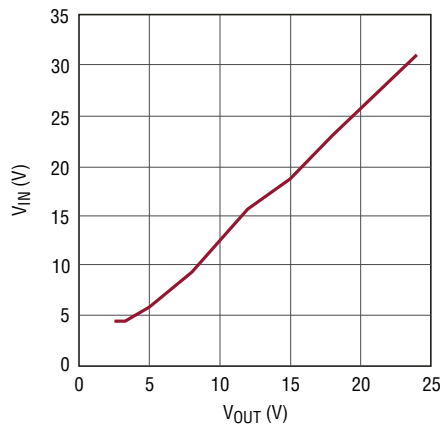
最小 V IN 与 V OUT 的关系曲线， I OUT = 4A
