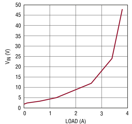
最小 V IN 与负载的关系曲线， V OUT = -12V
