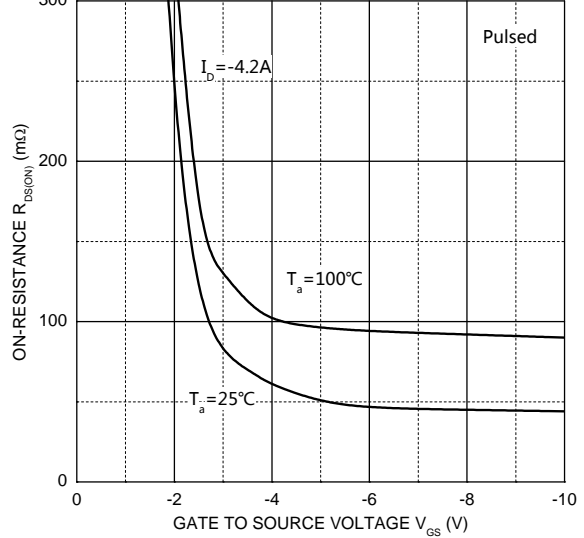
R_{DS(ON)} - V_{GS}
