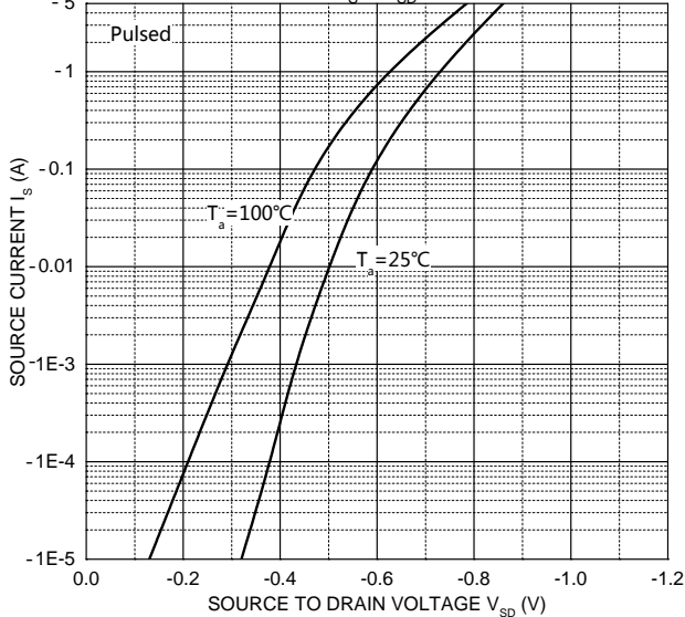
I_S - V_{SD}
