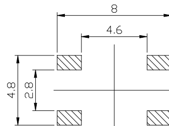
安装尺寸
