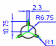
Reel dimensions
