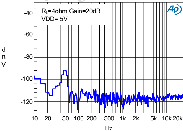
Noise FFT
