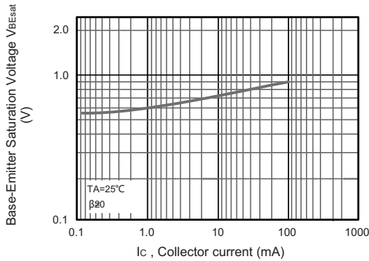
Fig.5 V_{BEsat}-I_C
