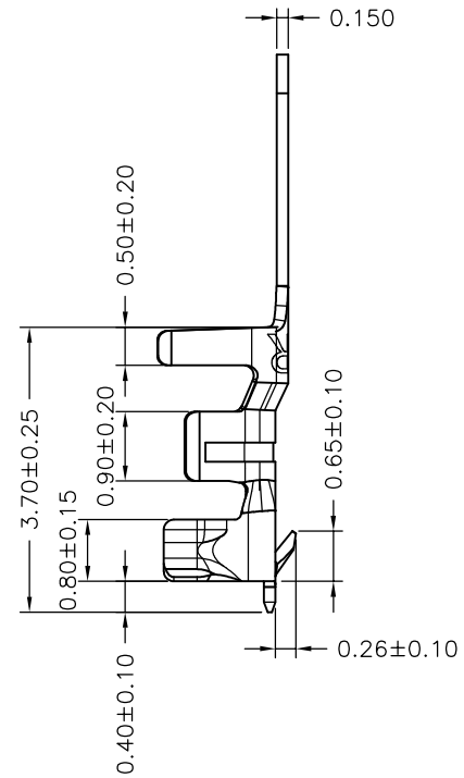
SEC:A-A
