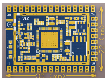
图 1 HLK-RM58S 封装大小
