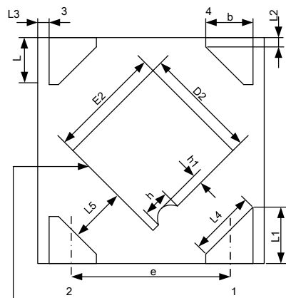
底视图
