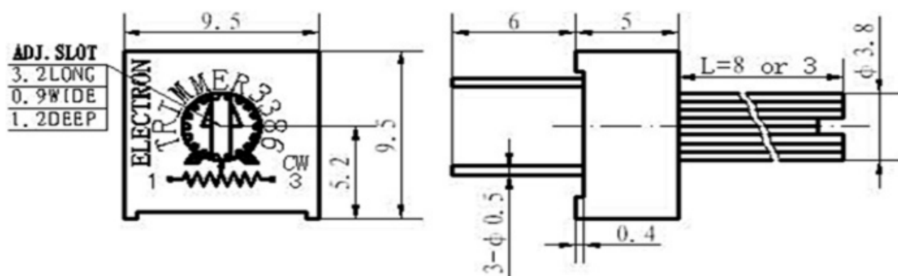
3386P型
